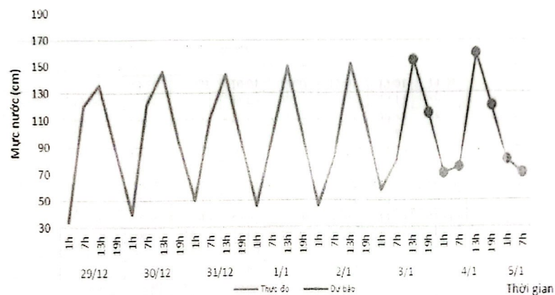
QUÁ TRÌNH MỨC NƯỚC THỰC ĐO VÀ DỰ BÁO TRẠM HÀ NỘI (SÔNG HỒNG)
